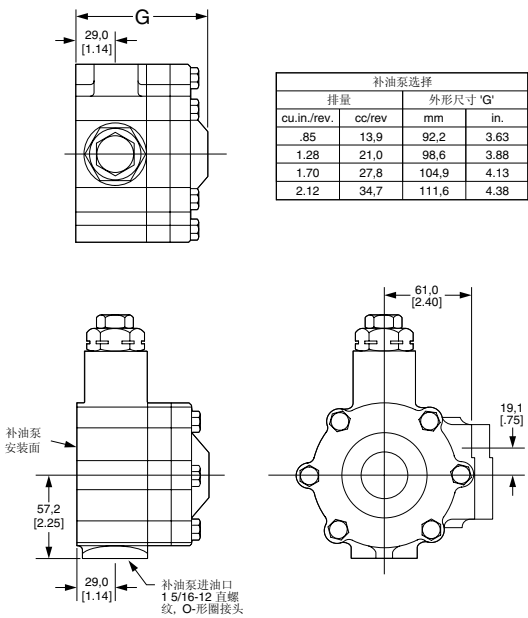
有 SAE B 辅助安装支口的补油泵
