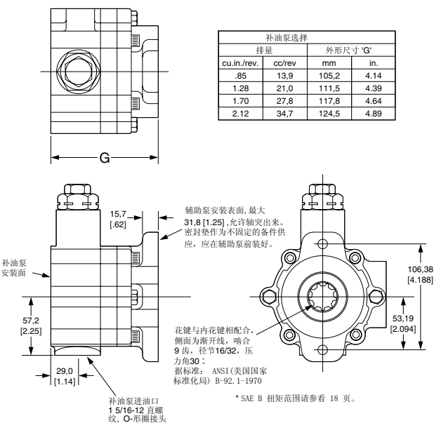
有远程滤油器接口的补油泵
