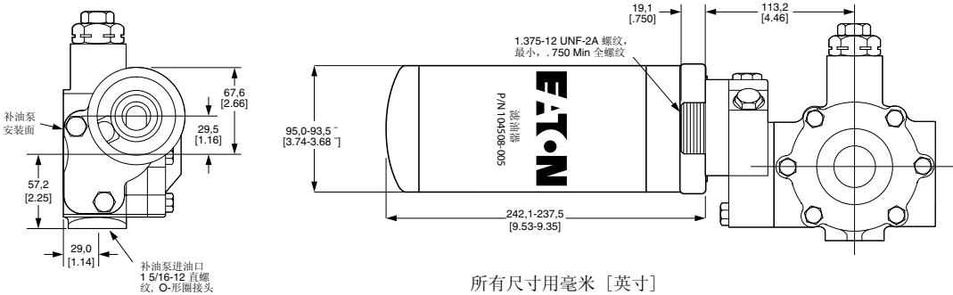
在边上带有一旋入式滤油器支口的补油泵
