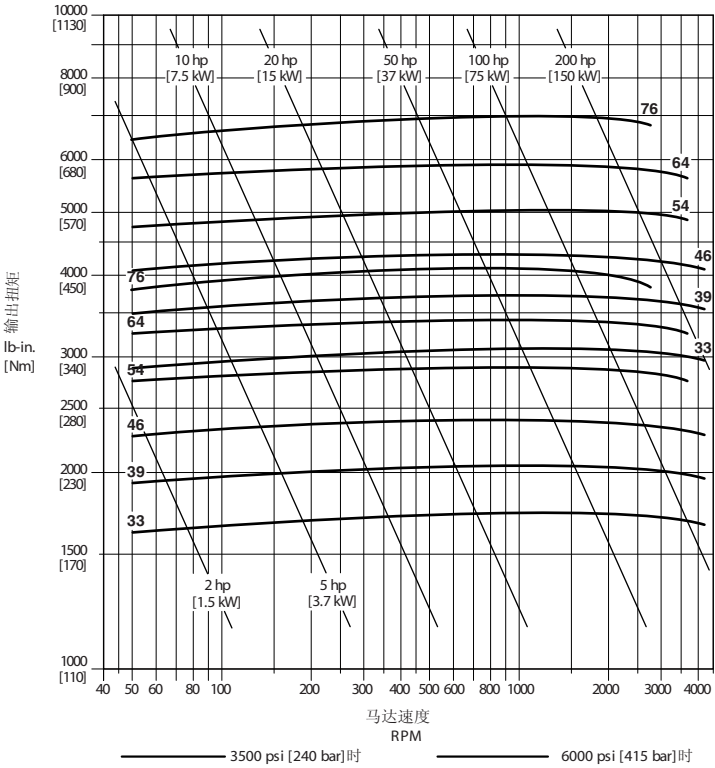
输出扭矩对速度
