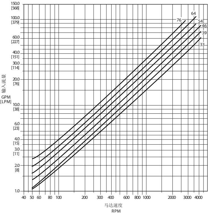
输入流量对速度
