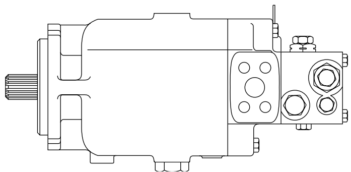
定量马达
