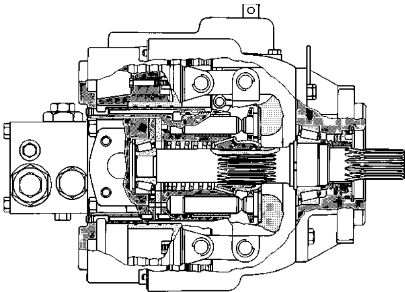
变量马达
