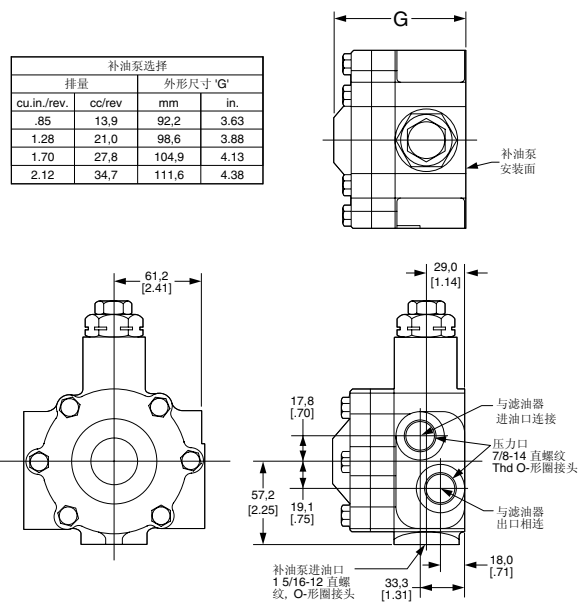
有远程滤油器接口的补油泵
