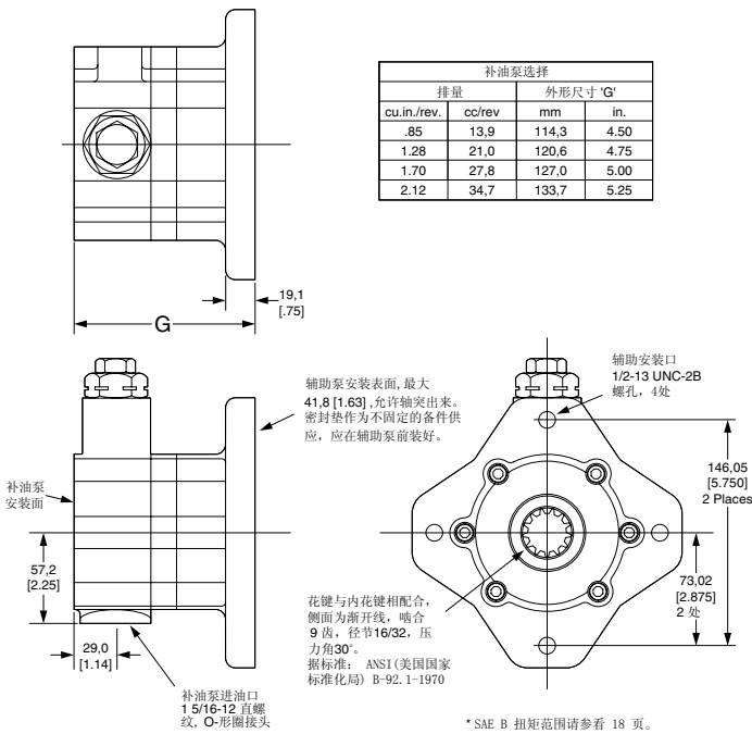
有 SAE B 辅助安装支口的补油泵
